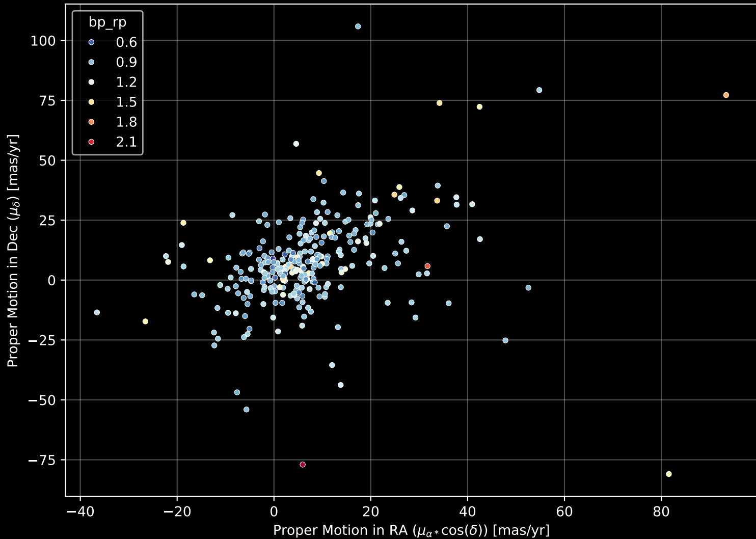
GALAH DR4 Field: [237] Proper Motion Diagram (n= 287)
