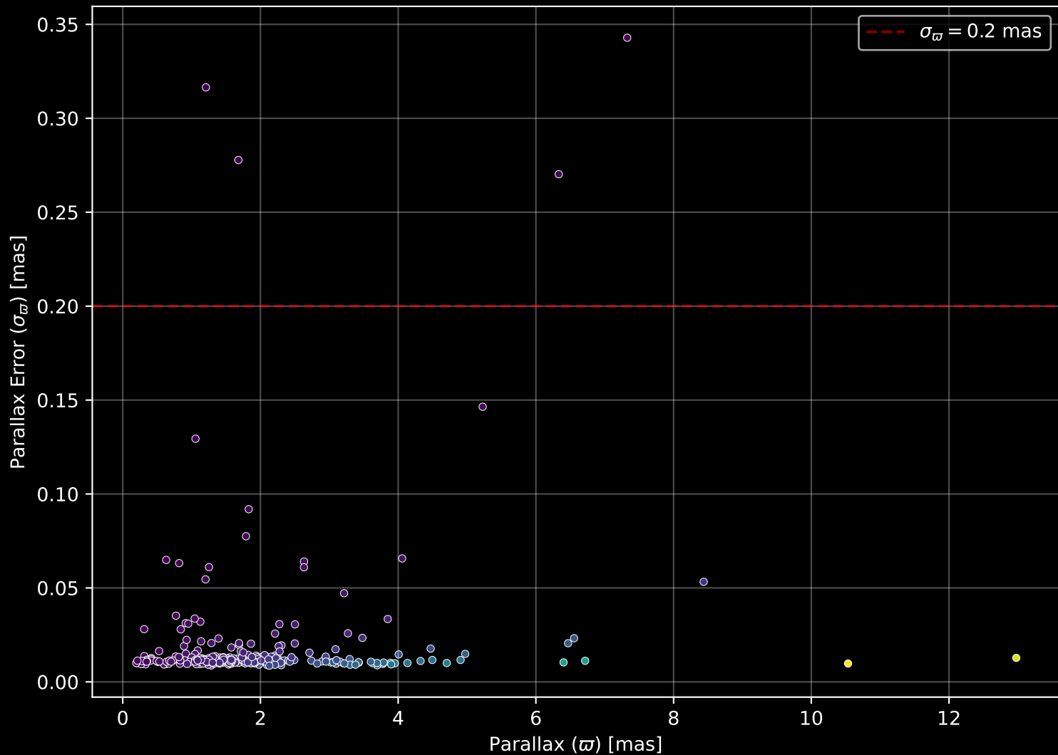
GALAH DR4 Field: [237] Parallax Quality (n= 287)
