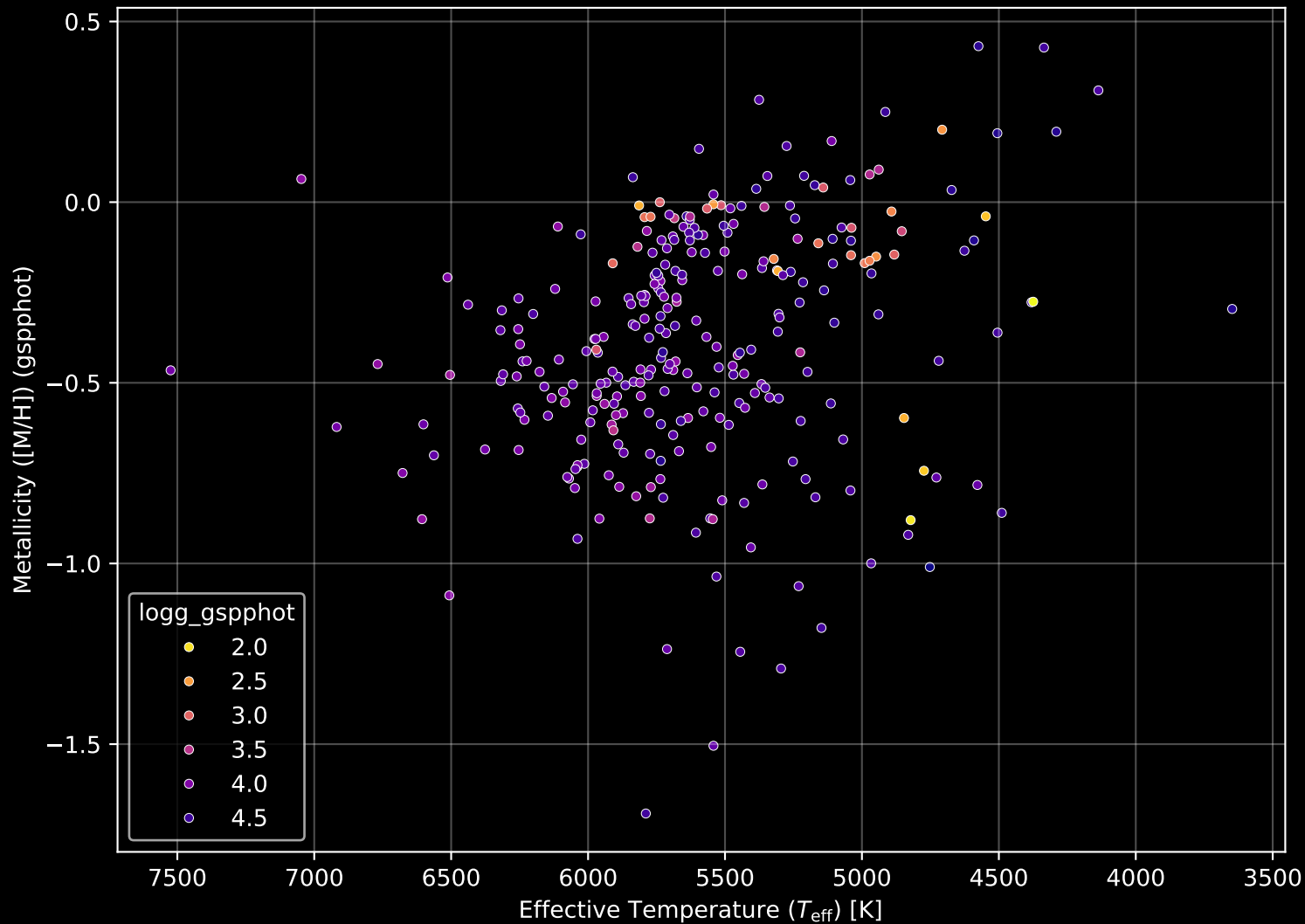
GALAH DR4 Field: [237] Stellar Population Parameters (n= 287)
