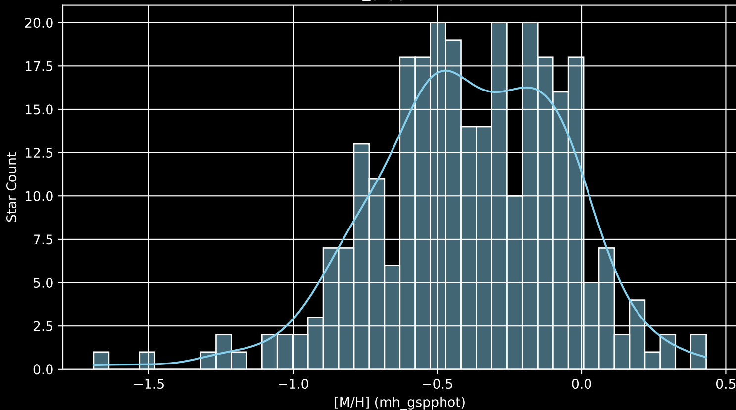
GALAH DR4 Field: [237] [M/H] (mh_gspphot) (n= 287)
